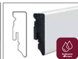
Battiscopa a incastro schiuma PS, impermeabile, adatto per locali soggetti a umidità, 15 x 50 mm 3
