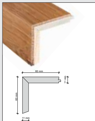
Bordi per chiusura scale con incastro unilaterale
