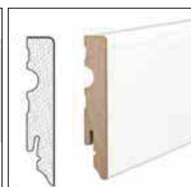
Battiscopa con rivestimento in pellicola MDF, 15x80 mm (cubo)
