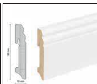
Profilo "Altdeutsch", battiscopa a incastro, cuore in legno massiccio verniciato, 18x96 mm
