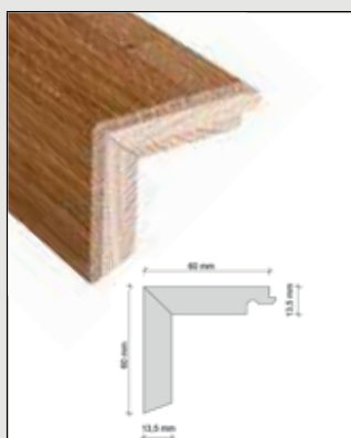
Listello per chiusura scale con incastro unilaterale
