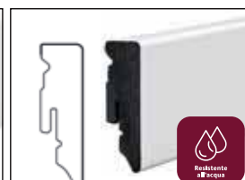
Battiscopa a incastro schiuma PS, impermeabile, adatto per locali soggetti a umidità, 15 x 50 mm (cubo)
