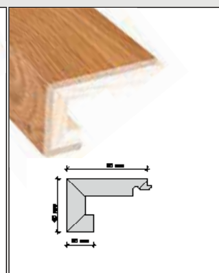
Listello per chiusura scale con incastro sui due lati
